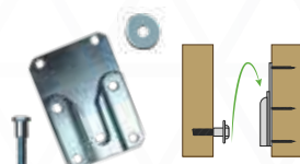
2169 Conector 3 piezas
